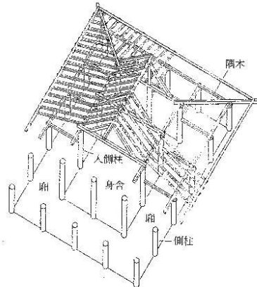
図 四面廂建物の基本構造
