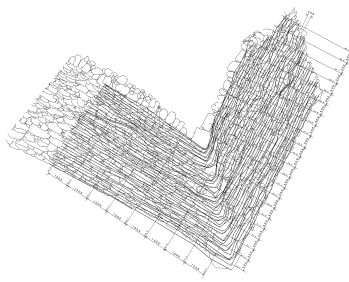
② 解体前に石垣の図面をとり、傾き等を調べ、復元のための資料を作ります。
