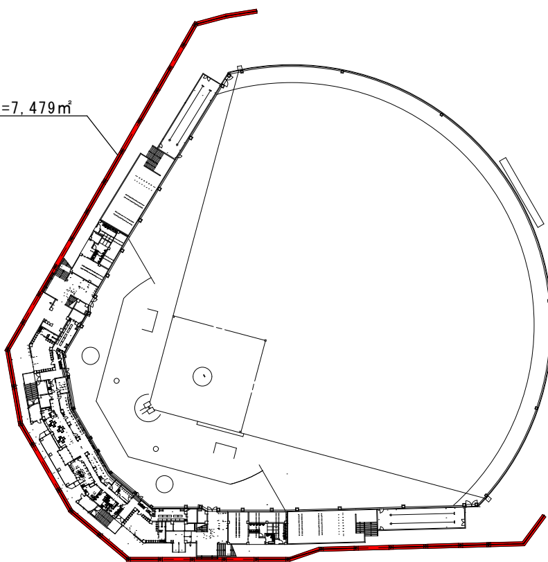
平面図
