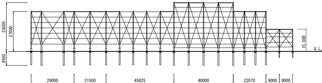
東側 立面図
