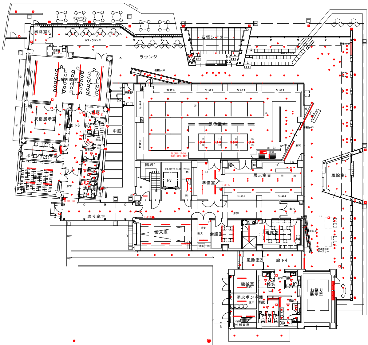
1階 照明設備平面図
