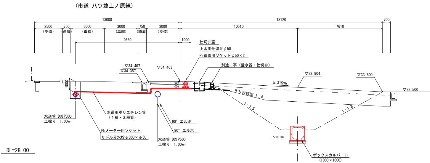
横断図
